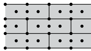
Rozmístění hmoždinek při počtu 10 ks na m 2
