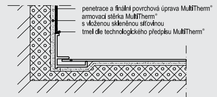
Podélný řez parapetem - lícovaný profil
