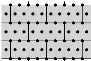
Rozmístění hmoždinek při počtu 14 ks na m 2
