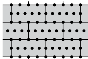
Rozmístění hmoždinek při počtu 16 ks na m 2
