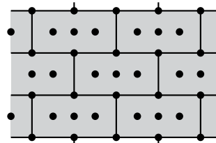
Rozmístění hmoždinek při počtu 10 ks na m 2
