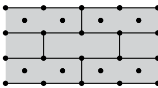
Rozmístění hmoždinek při počtu 6,5 ks na m 2
