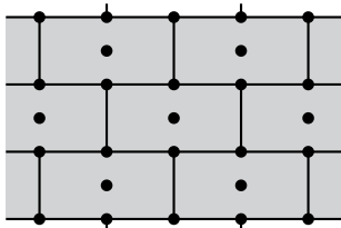
Rozmístění hmoždinek při počtu 6 ks na m 2
