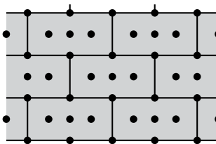
Rozmístění hmoždinek při počtu 8 ks na m 2
