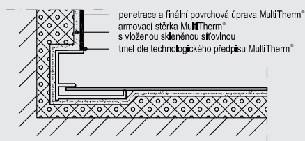
Podélný řez parapetem - zapuštěný profil
