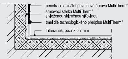
Podélný řez parapetem - A
