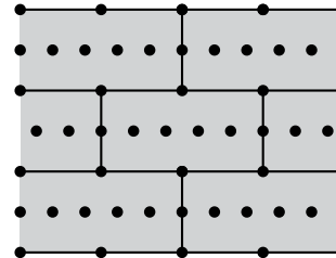
Rozmístění hmoždinek při počtu 10,8 ks na m 2
