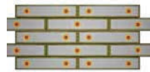
Rozmístění hmoždinek a lepidla při počtu 8 ks na m 2
