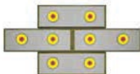
Rozmístění hmoždinek a lepidla při počtu 6 ks na m 2
