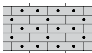
Rozmístění hmoždinek při počtu 8 ks na m 2
