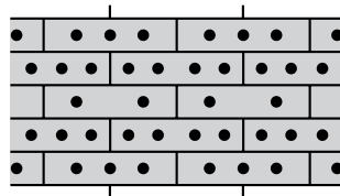
Rozmístění hmoždinek při počtu 16 ks na m 2
