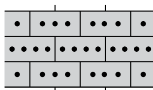
Rozmístění hmoždinek při počtu 10 ks na m 2
