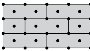
Rozmístění hmoždinek při počtu 8,8 ks na m 2
