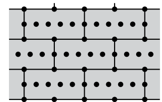
Rozmístění hmoždinek při počtu 12 ks na m 2
